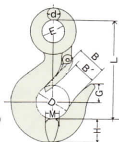
【新型重量フック 寸法表】 単位=m/m
