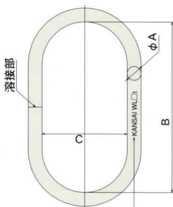
刻印 KANSAI WL□ t (□:使用荷重) PL (テスト荷重) = 使用荷重×2倍
