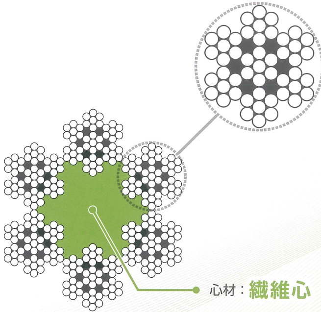
側ストランド構成 7×7
